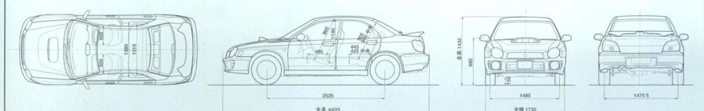
4面図(単位:mm) NB ※リヤスポイラー装着車
