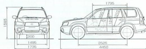
■4面図 単位:mm XT
