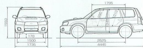
■4面図 単位:mm CROSS SPORTS
