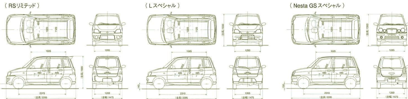
4面図 単位:mm
