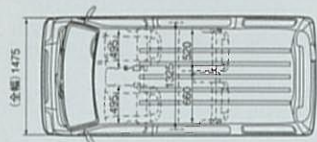
■寸法図(ディアスワゴンスーパーチャージャー) 単位=mm
