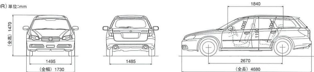
3面図(3.0R)単位:mm
