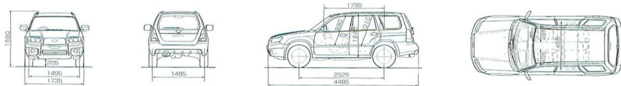
4面図(2.0X)単位:mm
